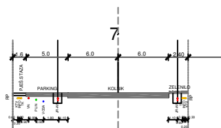
PROFILI 7 -10 VAN GRANICE OBUHVATA
