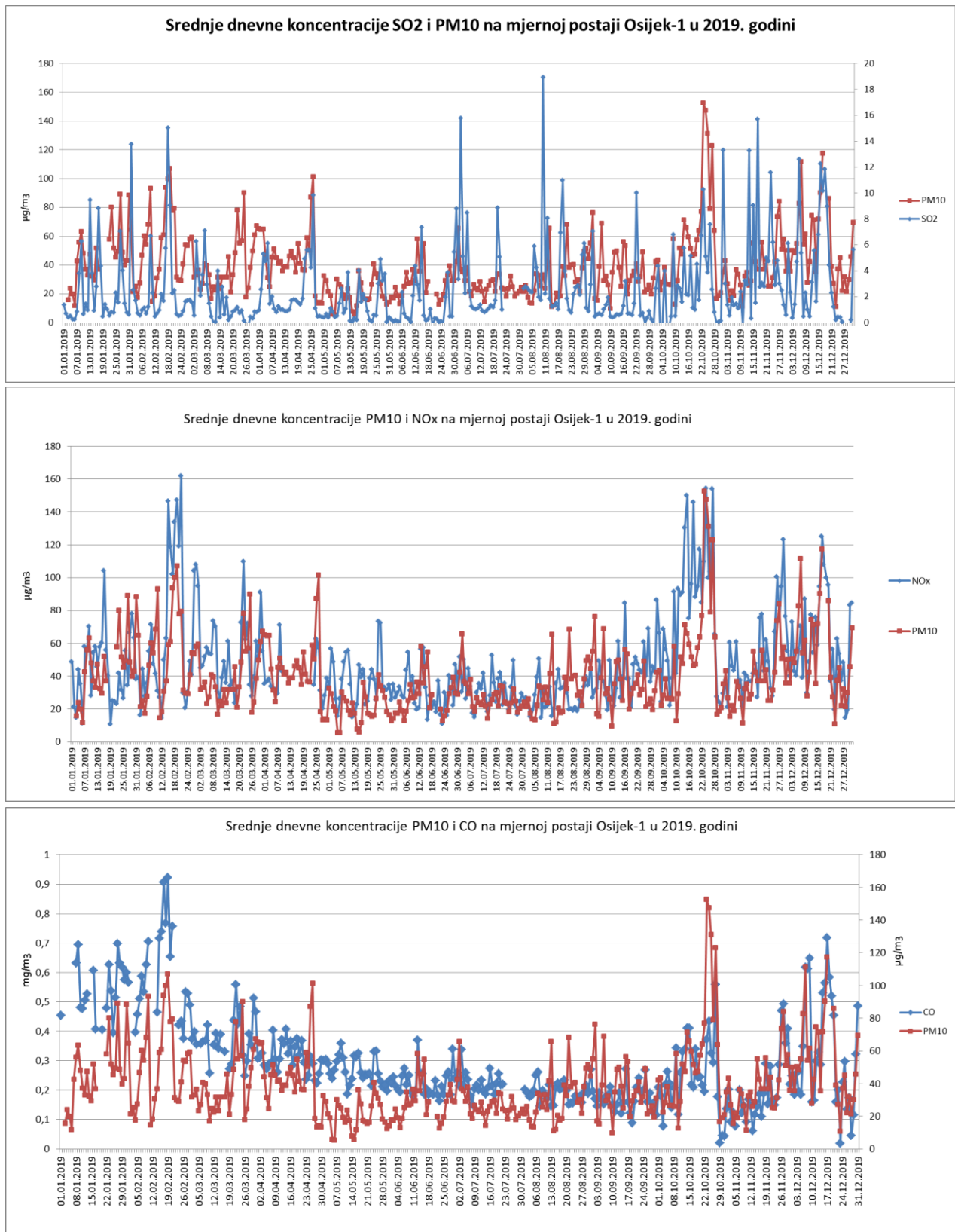
Slika 7.1-5. Trend srednjih dnevnih koncentracija lebdećih čestica PM 10 i NO 2 , PM 10 i CO na mjernoj postaji Osijek-1 2019. godine (Izvor: Baza podataka o kvaliteti zraka)
