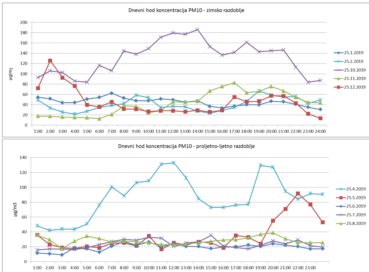
Slika 7.1-6. Dnevni hod koncentracija PM 10 na mjernoj postaji Osijek-1 2019. godine u zimskom i ljetnom razdoblju (Izvor: Baza podataka o kvaliteti zraka)
