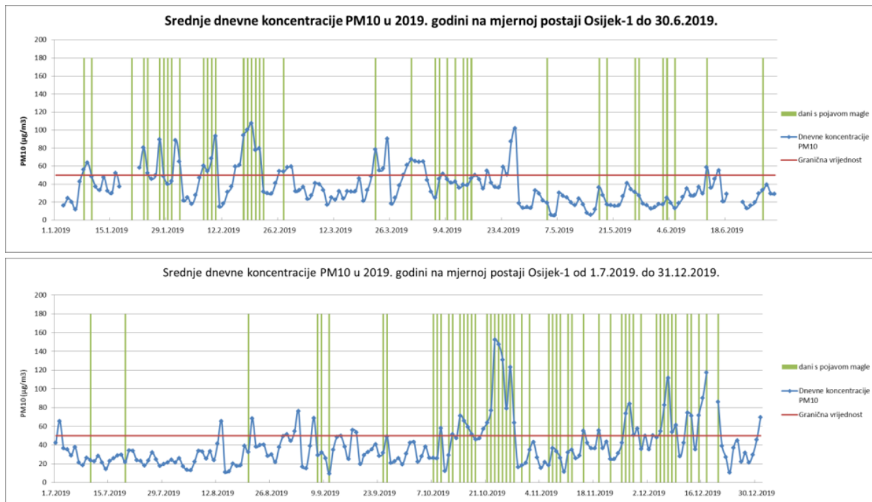
Slika 7.1-3. Srednje dnevne koncentracija PM_{10} na postaji Osijek-1 u 2019. godini i dani s pojavom magle na području Grada Osijeka (Izvor: Baza podataka o kvaliteti zraka, podaci s mjerne postaje Osijek-Čepin)
