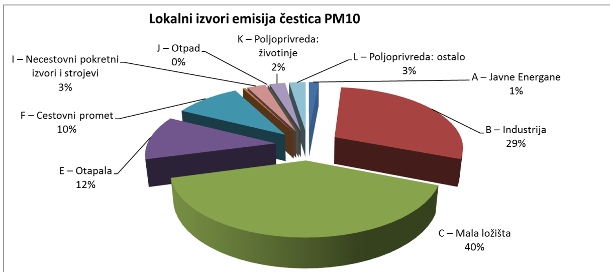
Slika 6.2-2. Raspodjela emisija PM 10 na području Grada Osijeka (Izvor: https://emep.haop.h , Obrada: Oikon d.o.o.)
