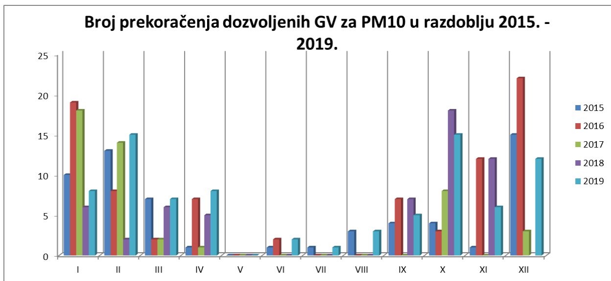
Slika 5.2-4. Kretanje broja prekoračenja GV lebdećih čestica PM 10 na mjernoj postaji Osijek-1 u razdoblju 2015.-2019. godine prema mjesecima (Izvor: baza Kvaliteta zraka u Republici Hrvatskoj http://iszz.azo.hr/iskzl Obrada: Oikon d.o.o.)
