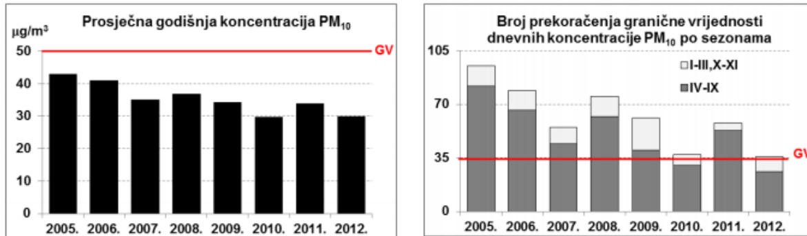
Slika 5.1-1. Prosječne godišnje koncentracije i broj prekoračenja dnevnih koncentracija PM 10 po sezonama na području Grada Osijeka u razdoblju 2005. – 2012. (Preuzeto: Akcijski plan smanjenja onečišćenja česticama (PM0) za Grad Osijek)
