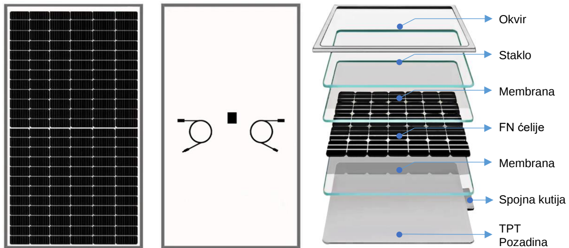
Slika 2.5-2 Fotonaponski panel
